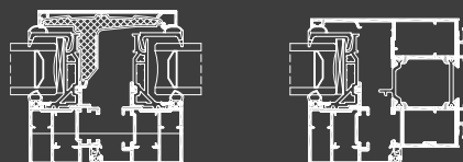
FENÊTRE 70 Ouvrant visible Série 5700 OF/OB à 1 ou 2 vtx
