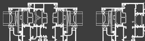
FENÊTRE 70 Ouvrant visible Série 5700 OF/OB à 1 ou 2 vtx
