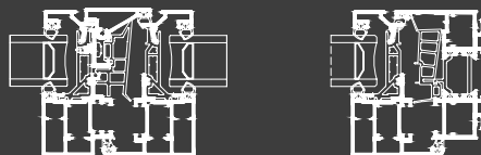
FENÊTRE 70 Ouvrant minimal Série 5700 OF/OB à 1 ou 2 vtx
