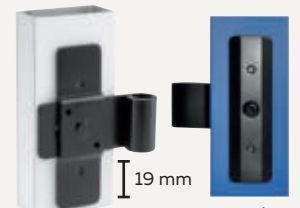
Équerre réglable EASY pour volets à cadre alu uniquement
